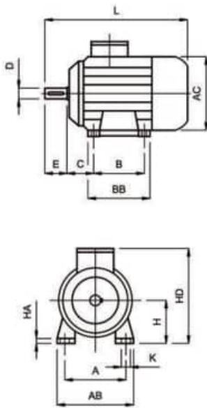
Motore su piedi IM 1081, IM B3 Motor on feet IM 1081, IM B3
