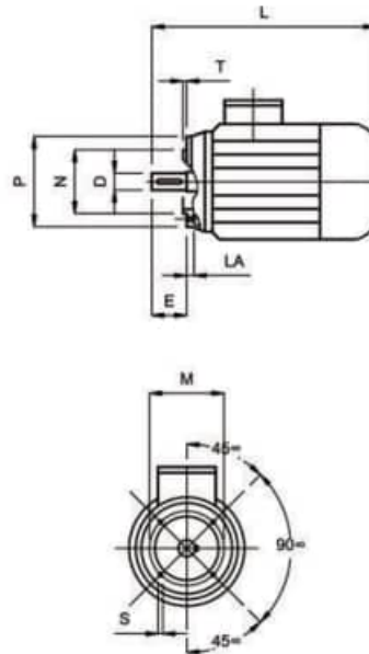
Motore con flangia piccola IM 3681, IM B14 Motor with small flange IM 3681, IM B14
