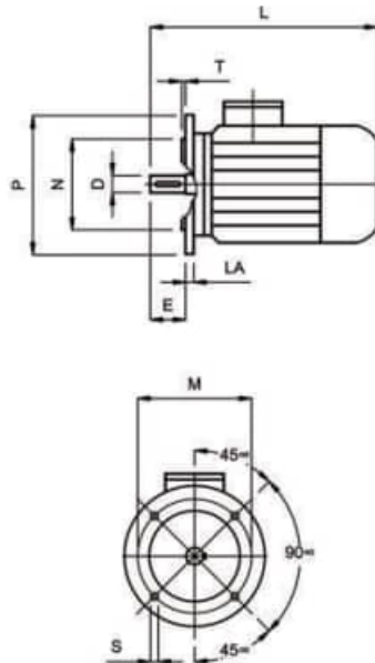
Motore con flangia grande IM 3081, IM B5 Motor with big flange IM 3081, IM B5
